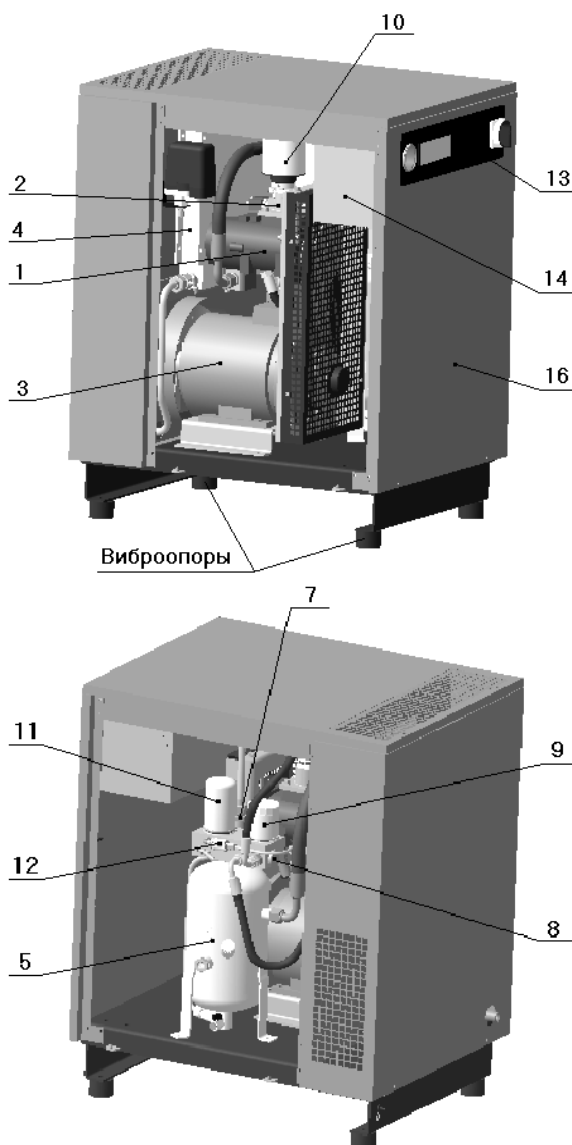
Рисунок 1 – Общий вид компрессорной установки BK5E-..., BK7E-..., BK10E-...
